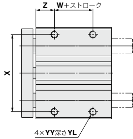
裏面図
