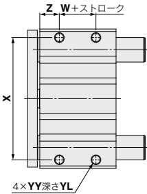
裏面図
